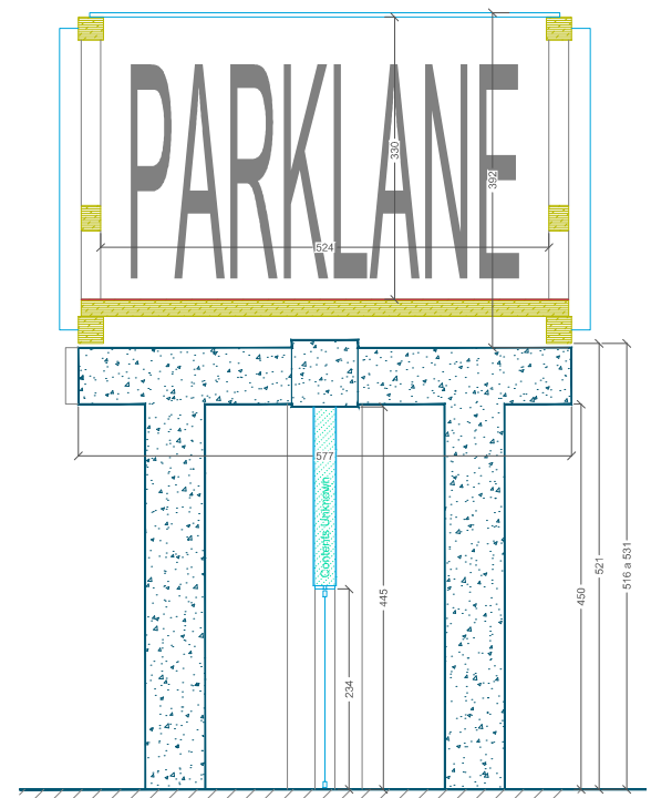
Section A-A 1/100
